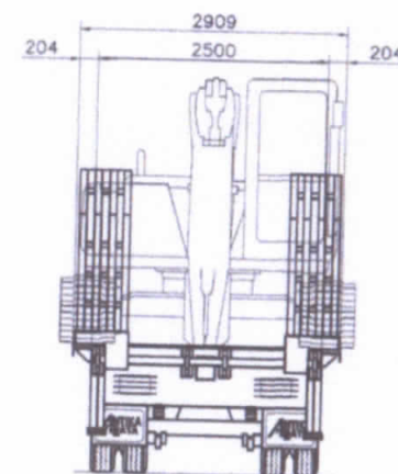
TAMPAK BELAKANG
